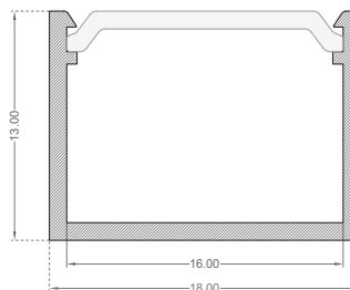
sol.p18rect13.s16
